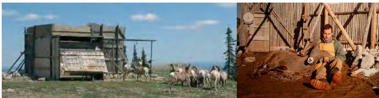
Figura 8.17: Impianto di cattura fisso per la cattura di big horn sulle Montagne Rocciose dell'Alberta in Canada attirati dal sale. La struttura è dotata di portone basculante con comando remoto (foto: Nicoloso)
