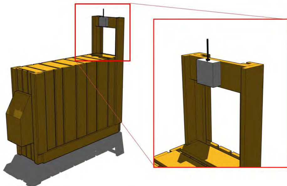
Figura 8.6: rendering di una trappola a cassetta dotata di dispositivo di scatto elettronico e comunicazione di avvenuta chiusura con SMS (Disegni. Nicoloso S.)
